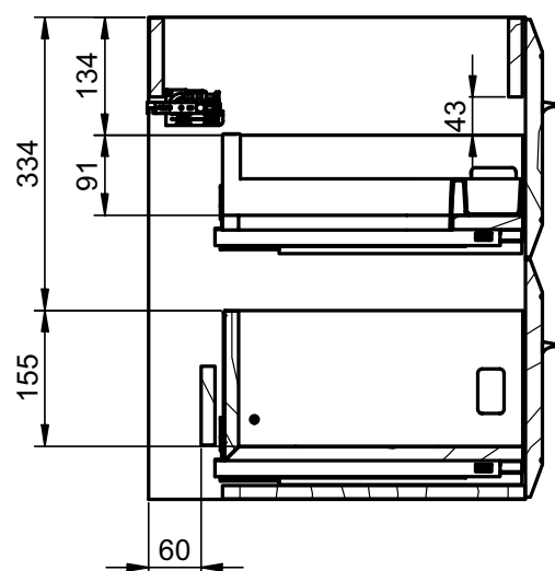
B-B ( 1 : 8 )
