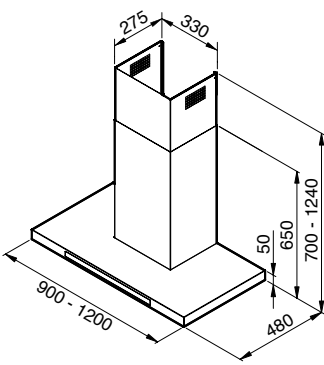
Planos dimensionales y de instalación.
