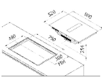
Instalación sobrepuesta
