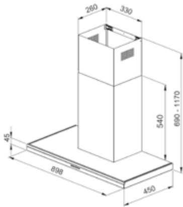
Planos dimensionales y de instalación.
