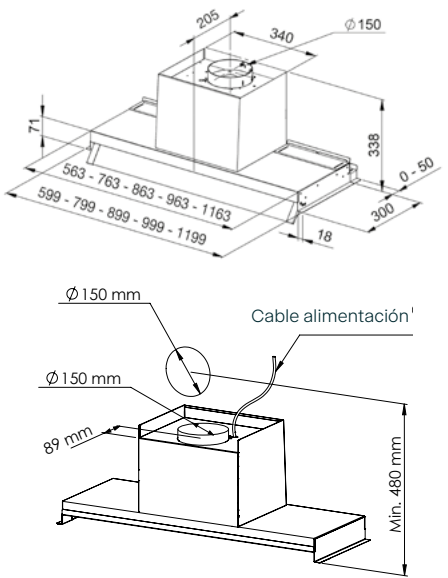
Planos dimensionales y de instalación. Datos medidos conforme a normas UNE-EN 61591 y UNE-EN 60704
