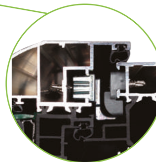
Conçu pour conserver la compression sur la hauteur de l'ouvrant
