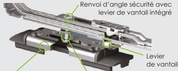
Renvoi d'angle sécurisé en partie haute
