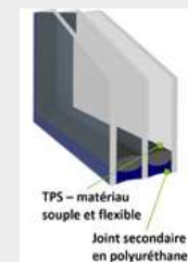
Coupe de l'intercalaire TPS
