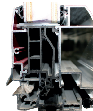
Excellente étanchéité à l'air, à l'eau et au vent grâce au joint central et à la rupture thermique.
