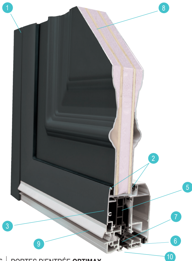
Seuil à rupture de pont thermique PMR gris anodisé
