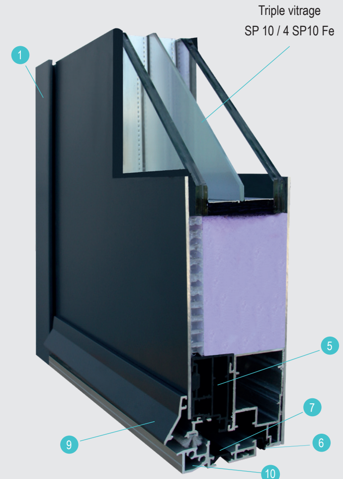
Excellente étanchéité à l'air, à l'eau et au vent grâce au joint central et à la rupture thermique.
