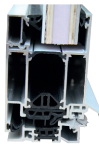
Excellente étanchéité à l'air, à l'eau et au vent grâce au joint central
