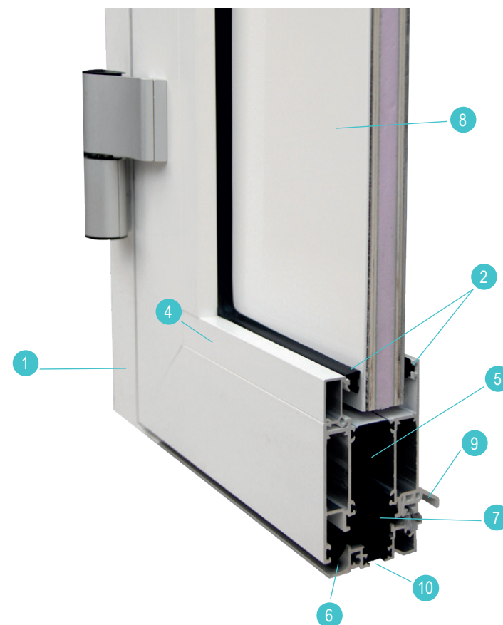
Excellente étanchéité à l'air, à l'eau et au vent grâce au joint central
