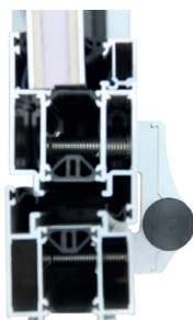
Les vis traversent 2 parois d'aluminium
