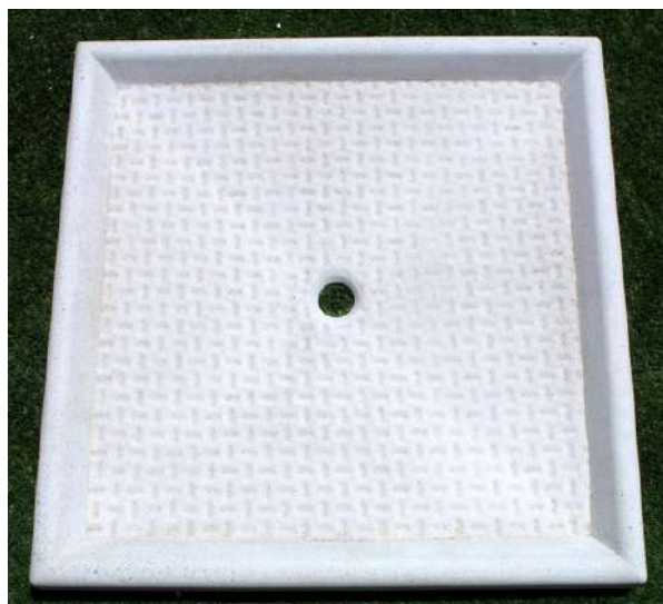
Modelo Rejilla 80cmx80cmx7desagüe de 4 70xcmx70cm desagüe del 6
