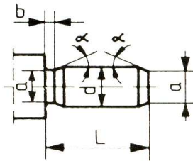
Gewindezapfen
