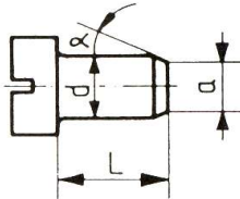
Kopfschraube ohne Schaft
