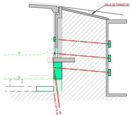
Abaissement culée Est pont Haut de Crans
