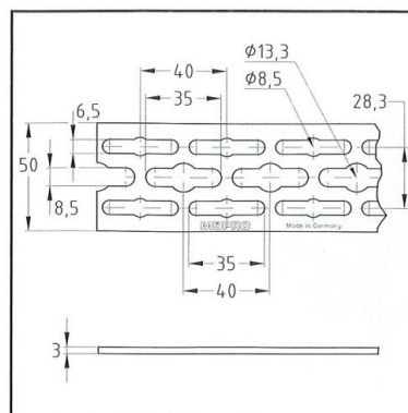
StaboFix® Schiene
