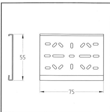
StaboFix® Halteblech
