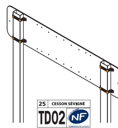
Fixation directe sur panneau Prévoir supports et brides
