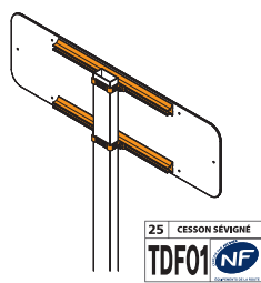
Fixation rails au dos Prévoir support et brides
