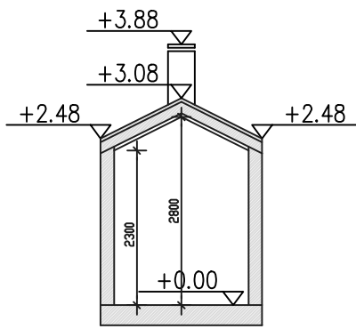
LEIKKAUS A-A
