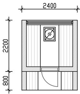
POHJAPIIRROS / SAUNA 2
