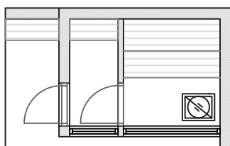
POHJAPIIRROS / SAUNA 1
