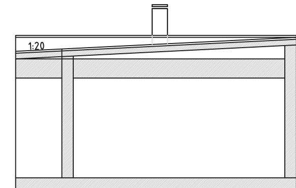
LEIKKAUS A-A
