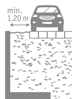
A | Verkehrslast bis p = 5 \text{ kN/m}^2 ohne Anpralllasten, Abstand: 1,2 m (bis 155 cm Höhe)/1,5 m (ab 180 cm Höhe)
