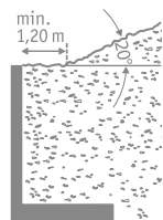
B | Böschung Ge- ländeneigung 20°, Verkehrslast bis p = 5 \text{ kN/m}^2 , Abstand: 1,2 m (bis 155 cm Höhe)/1,5 m (ab 180 cm Höhe)
