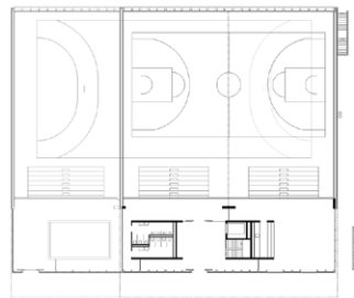
Plan du rez-de-chaussée
