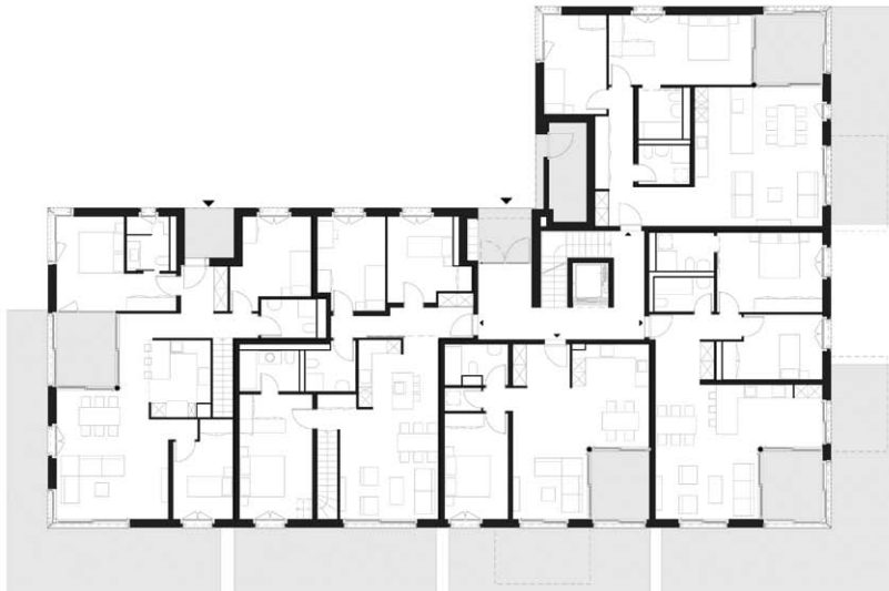
Rez-de-chaussée
