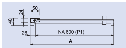
Dibujo técnico NA520
