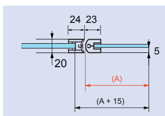
Datos técnicos VI525
