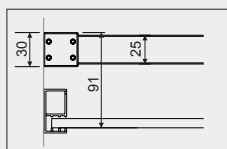
Detalle fijación barra a pared
