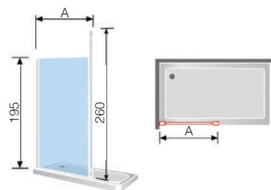
Dibujo técnico FL633 Panel Fijo de Ducha a Techo
