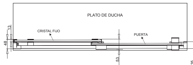
Dibujo técnico VO102 Frente de Ducha sin perfil de cierre
