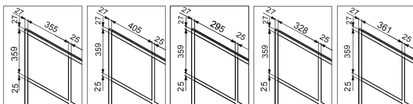
Detalle decorado Panel de 80 cm
