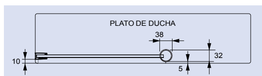
Dibujo técnico FL633 Panel Fijo de Ducha a Techo
