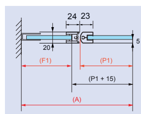
Detalle datos técnicos PL524
