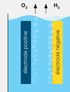
Système ouvert, batterie plomb-acide
