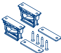
Ref. 32703SA Kit 2 suplementos hoja fija Domo 125/125R
