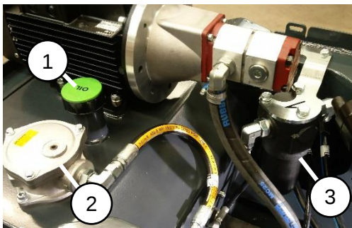
Kuva 22: Hydraulioöljynsuodattimen sijainti
