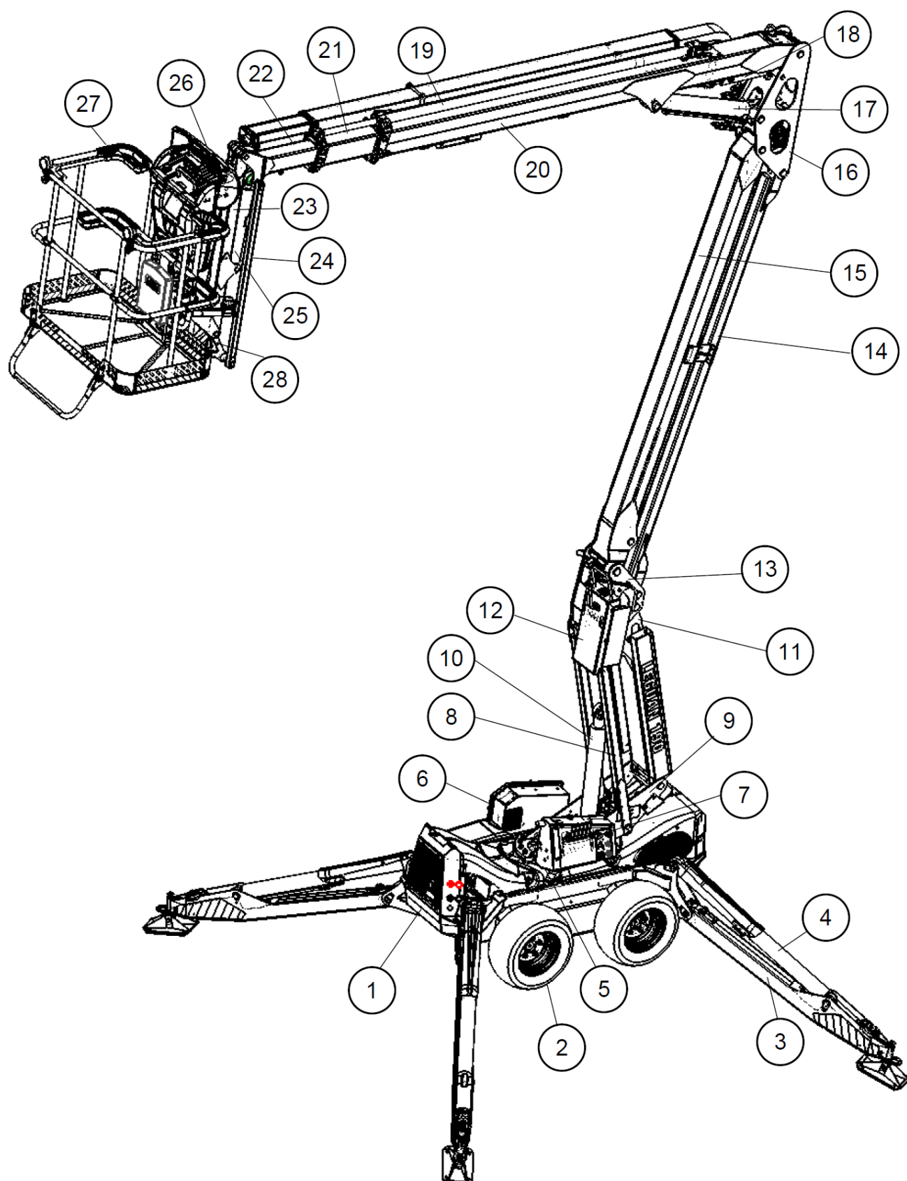
Kuva 1 Nostimen komponentit
