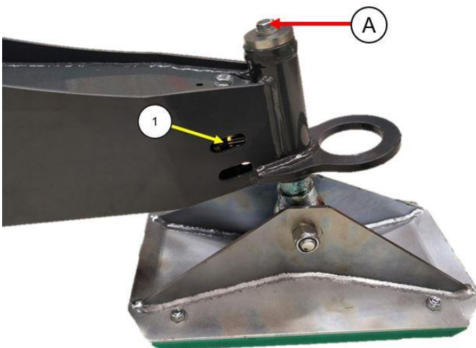
Kuva 19 Tukijalan anturointi (1) ja tunnistustapin lukitus (A)
