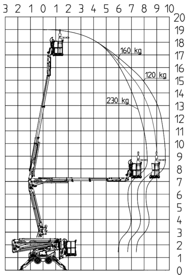
Kuva 3 Ulottumakaavio
