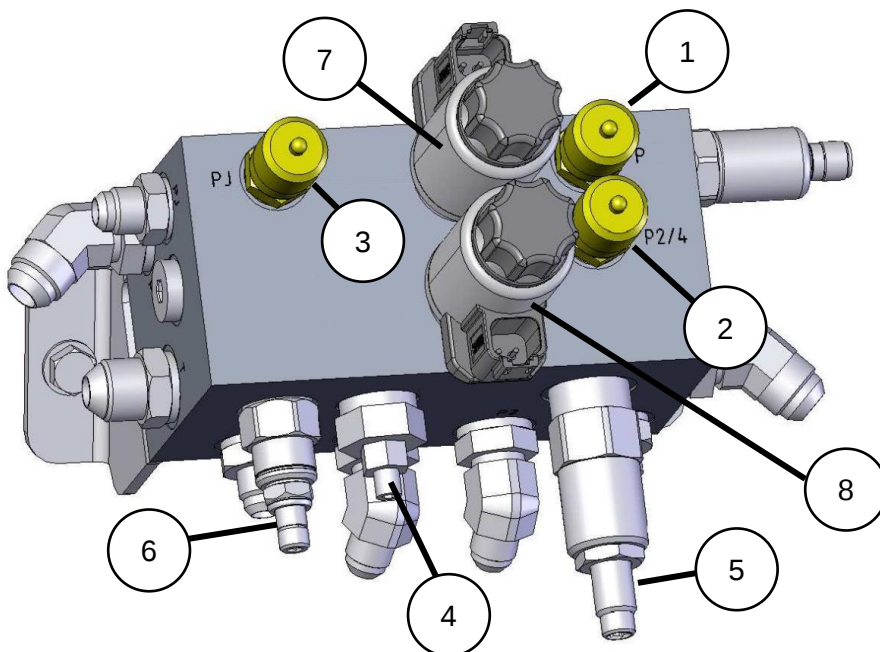
Kuva 26: Pumppulohko
