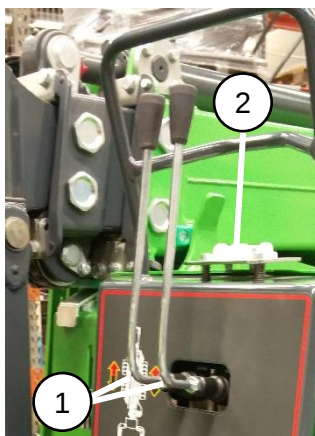
Kuva 10: Siirtoajon ohjausvivut
