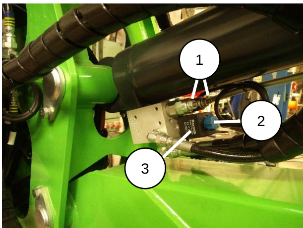
Kuva 28 Taittosylinderi
