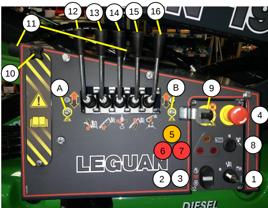
Kuva 6: Alaohjauspaneeli
