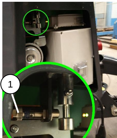
Kuva 30: Alempi kuljetustuen anturi
