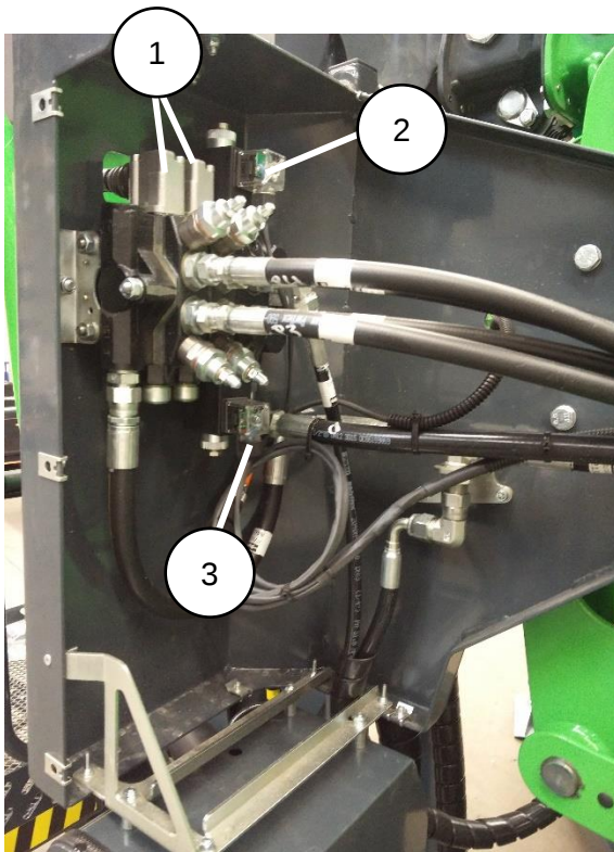
Kuva 27: Jalustan venttiilikotelo
