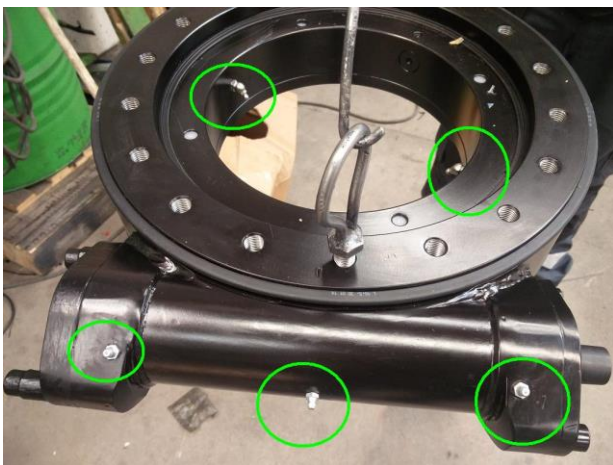
Kuva 15: Kääntökehän voitelupisteet, kehä kuvattuna yläpuolelta
