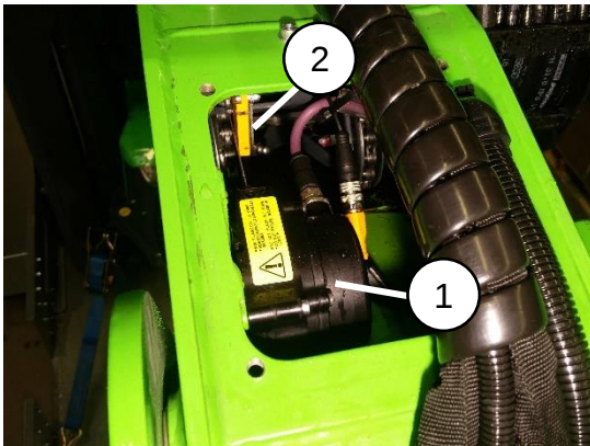
Kuva 33: Taittopuomin anturointi
