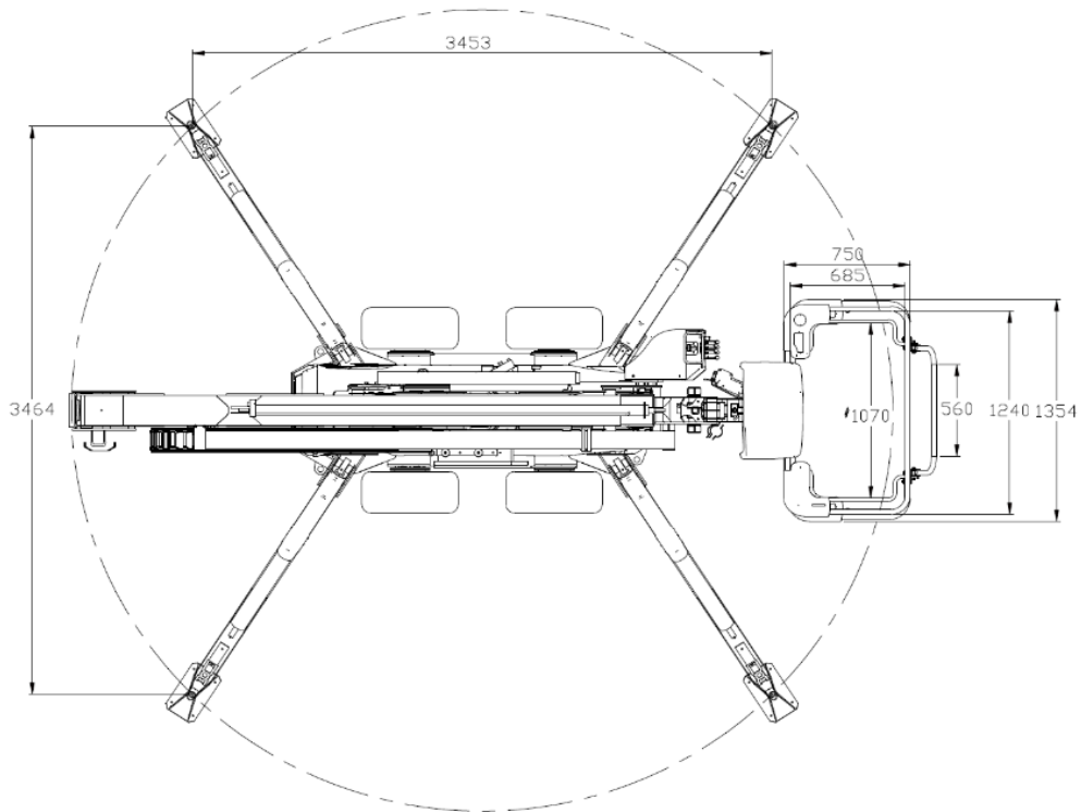
Kuva 2 Työaluekaavio
