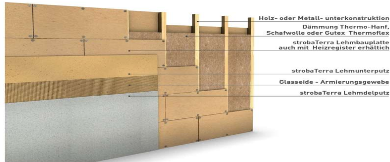
AUFBAU EINER LEICHTBAUWAND BEIDSEITIG BEPLANKT
