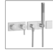
HANSADESIGNO Fertigmontage-Installationspaket 3.2 Einhand-Batterie, DN 15 (G1/2) passend zu HANSAMATRIX Einbaukörper* 4487 0130 verchromt mit Brause-Set, für entfernt liegenden Wanneneinlauf (HANSAFILL)
