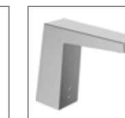
HANSALOFT Waschtisch-Elektronik-Batterie, DN 15 Netzbetrieb (inkl. Netzteil) 5749 2211 verchromt berührungslos elektronisch gesteuert (Infrarot), mit Ablaufgarnitur (Metall) Ausladung: 143 mm
