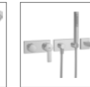
HANSA LIVING Fertigmontage- Installationspaket 1.3 Einhand-Batterie, DN 15 (G1/2) passend zu HANSAMATRIX Einbaukörper* 4487 1100 verchromt mit Brause-Set, mit Wanneneinlauf, DN 15
