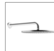
HANSAVIVA Kopfbrause, DN 15 4426 0300 verchromt Brausekopf, Messing Ø 300 mm Ausladung: 357 mm
