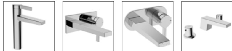
HANSALOFT Waschtisch-Einhand-Einloch-Batterie, DN 15 5756 2103 verchromt für flache Aufsatzwaschbecken, ohne Ablaufgarnitur, Anschluss über Kupferrohre Ausladung: 114 mm HANSALOFT Fertigmontageset Waschtisch-Einhand-Wand-Batterie, DN 15* 5757 2103 verchromt Ausladung: 197 mm HANSALOFT Fertigmontageset Waschtisch-Einhand-Wand-Batterie, DN 15* 5757 2103 verchromt Ausladung: 193 mm HANSALOFT Waschtisch-Dreiloch-Batterie, DN 15* 5768 2103 verchromt incl. Push-Ablaufgarnitur Ausladung: 141 mm
