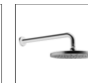
HANSAVIVA Kopfbrause, DN 15 4426 0100 verchromt Brausekopf, Messing Ø 202 mm Ausladung: 357 mm
