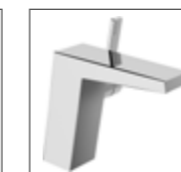
HANSALOFT Waschtisch-Einhand-Einlochbatterie, DN 15 5752 2203 verchromt ohne Ablaufgarnitur, Anschluss mit flexiblen Druckschläuchen Ausladung: 146 mm
