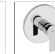
HANSA LIVING Fertigmontageset mit Funktionseinheit Einhand-Brause-Batterie passend zu HANSABUEBOX Einbaukörper* 8387 9503 verchromt schraubenlose Rosette, Rosette rund, Ø 170 mm, Funktionseinheit ohne Umstellung
