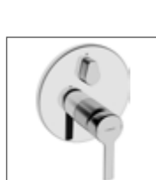
HANSA RONDA Fertigmontageset mit Funktionseinheit Einhand-Wannen-Batterie mit Sicherungseinrichtung passend zu HANSABLUEBOX Einbaukörper* 8384 3573 verchromt schraubenlose Rosette, Rosette rund, Ø 170 mm, Funktionseinheit mit BLUESWITCH Umstellung
