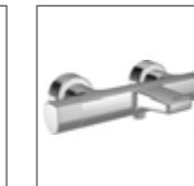
HANSAEMPRA STYLE Wannen-Thermostat-Batterie, DN 15 (G 1/2) 5844 2101 verchromt Ausladung: 159 mm
