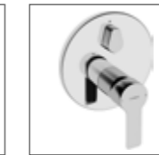
HANSA LIVING Fertigmontageset mit Funktionseinheit Einhand-Wannen-Batterie passend zu HANSABUEBOX Einbaukörper* 8385 9503 verchromt schraubenlose Rosette, Rosette rund, Ø 170 mm, Funktionseinheit mit BLUESWITCH Umstellung
