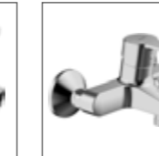
HANSAPRIMO Einhand-Wannen-Batterie, DN 15 (G 1/2) 4944 2103 verchromt Ausladung: 155 mm
