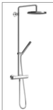
HANSATEMPRA STYLE Brause-Thermostat-Batterie, DN 15 (G 1/2) 5842 9103 verchromt mit direkt angeschlossenem Duschsystem, Brausekopf, Messing Ø 220 mm, HANSASTILO-Handbrause, 1-strahlig
