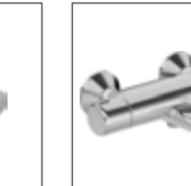
HANSAMICRA Wannen-Thermostat- Batterie, DN 15 (G 1/2) 5816 2171 verchromt THERMO COOL-Funktion Ausladung: 159 mm
