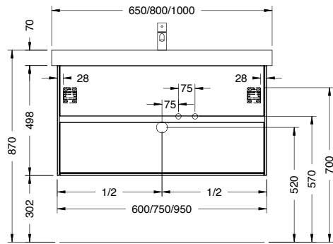
Villeroy&Boch Subway 2.0 WU341/ 342/ 343
