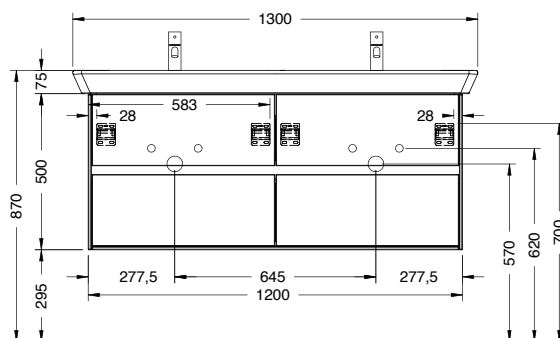
Vitra T4 WU354
