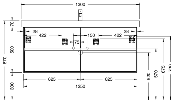
Villeroy&Boch Subway 2.0 WU345
