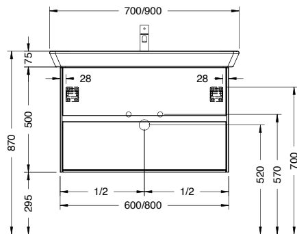
Vitra T4 WU354
