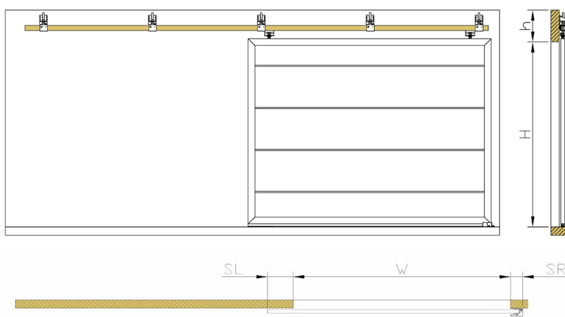
Sivulukko tai lattialukko saatavana pyynnöstä
