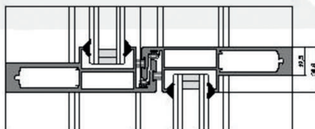
CRUCE REFORZADO
