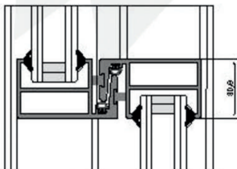
CRUCE SIMPLE
