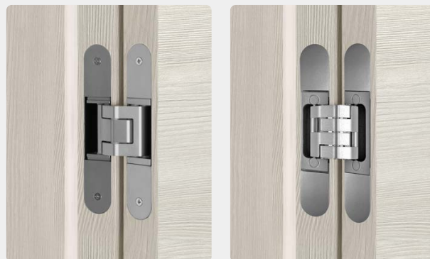
Das verdeckt liegende Band ist bei stumpfen Türen die erste Wahl, da es bei geschlossener Tür nicht sichtbar ist. »Tectus« Band TE 340 3D links, »Pivota« Band DX 61 3-D Design, rechts
