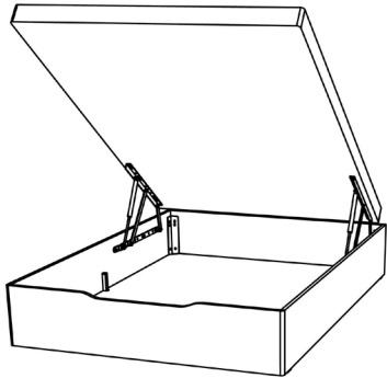
Coffre Optimo ouvert
