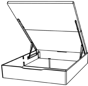
Coffre Maximo option scindable
