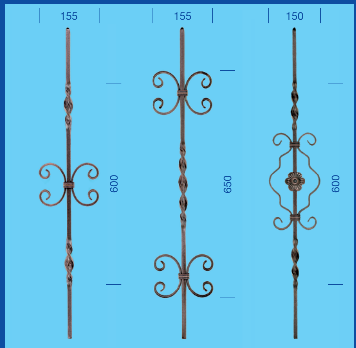
Art.-Nr. 12500 12 × 12 mm glatt 1,4 kg
