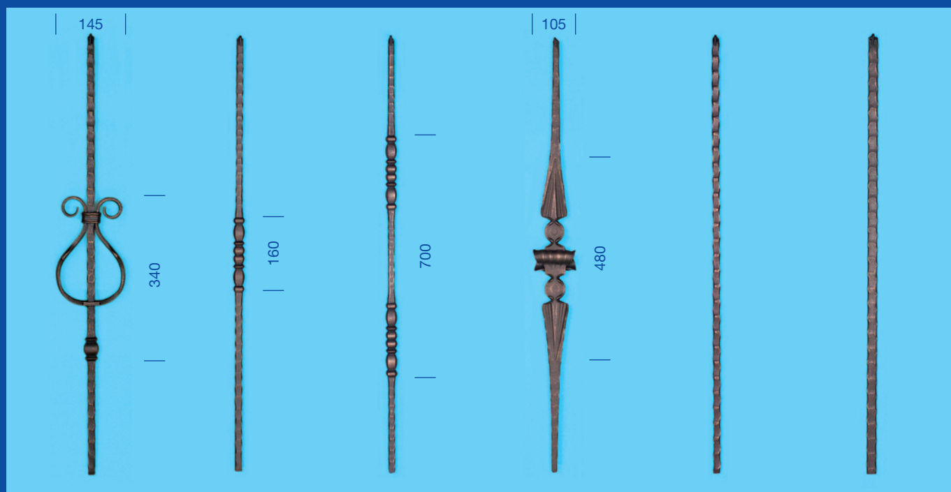
Art.-Nr. 10780 14 × 14 mm 2,6 kg
