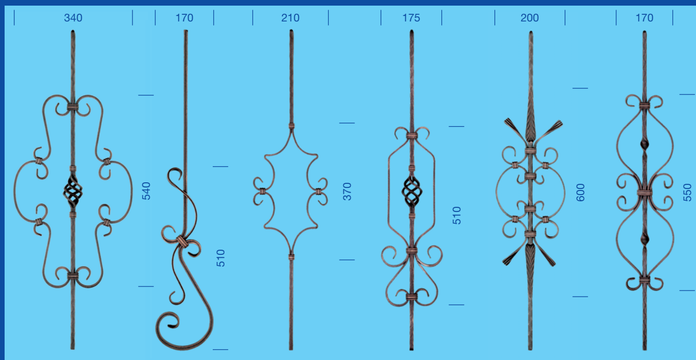
Art.-Nr. 12530 12 × 12 mm 2,7 kg
