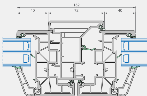
Elegant ThermoFibra Infinity 115 X horizontaal
