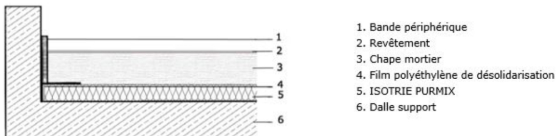
Figure 2 : Désolidarisation périphérique
