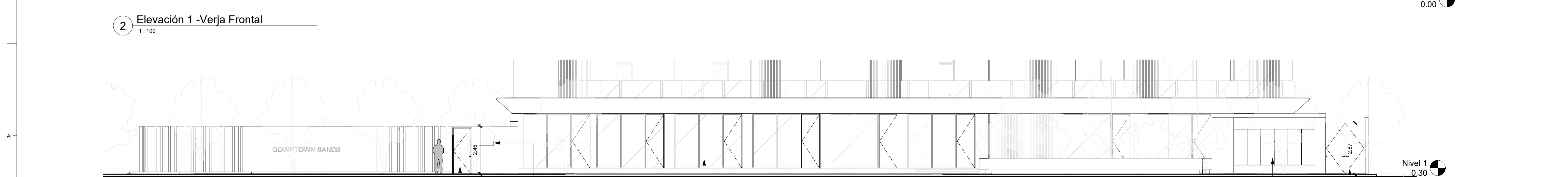
3 Elevación 2 - Verja Frontal 1:100
