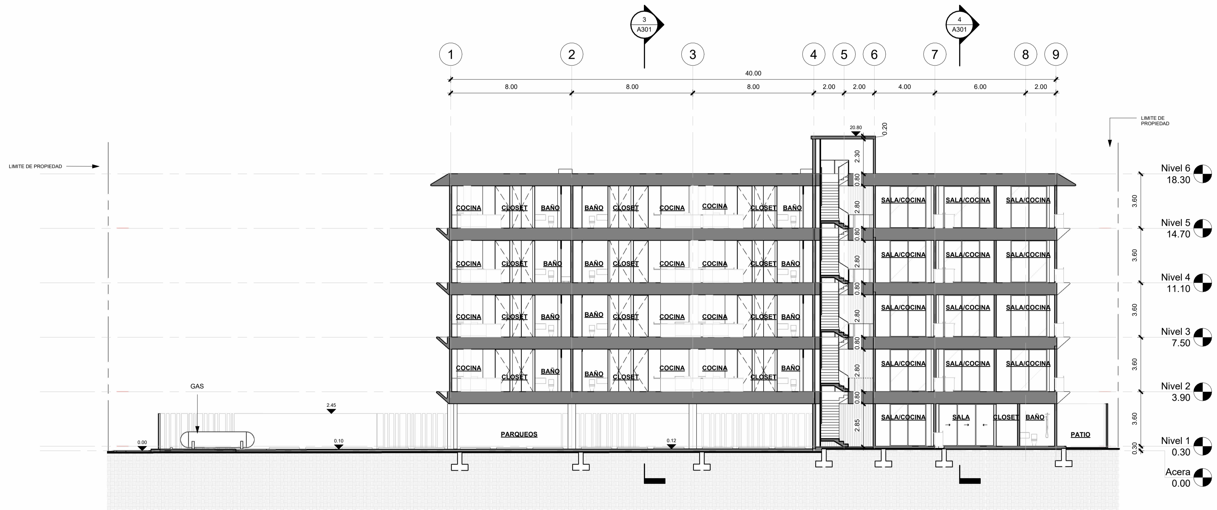
2 Seccion 2 1 : 150
