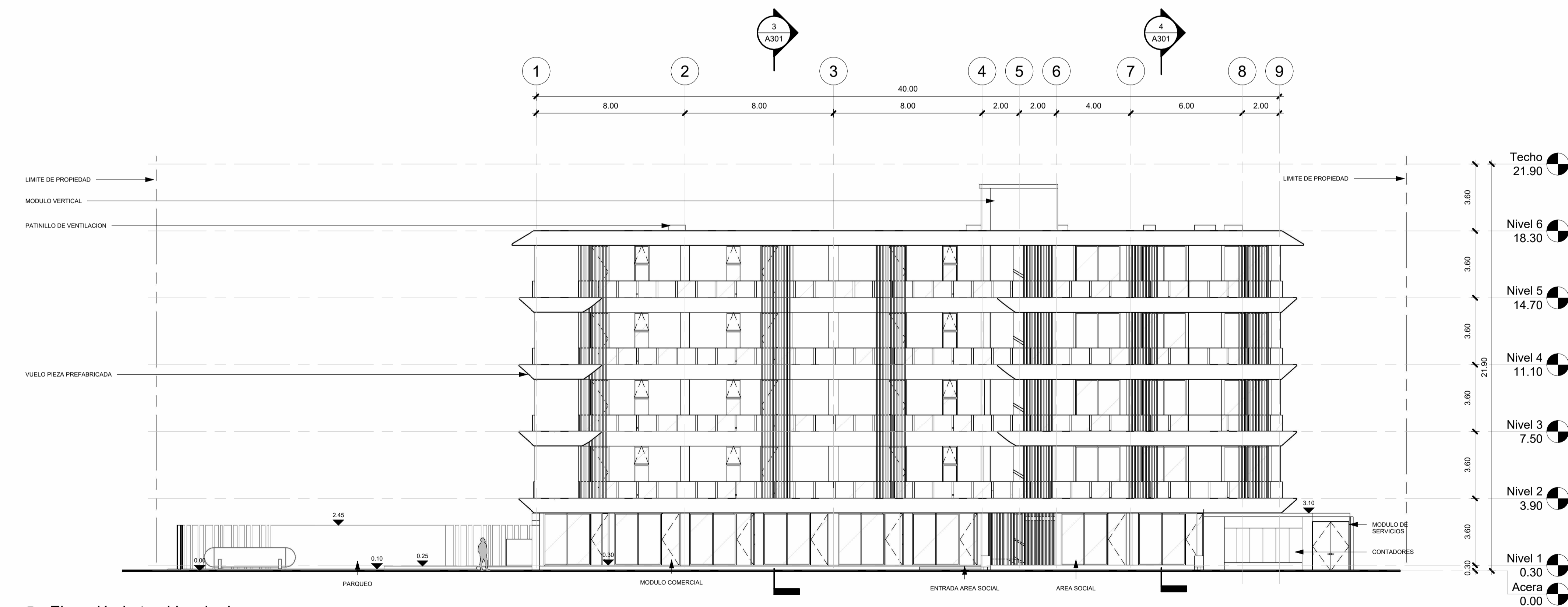
2 Elevación Lateral Izquierdo 1 : 150
