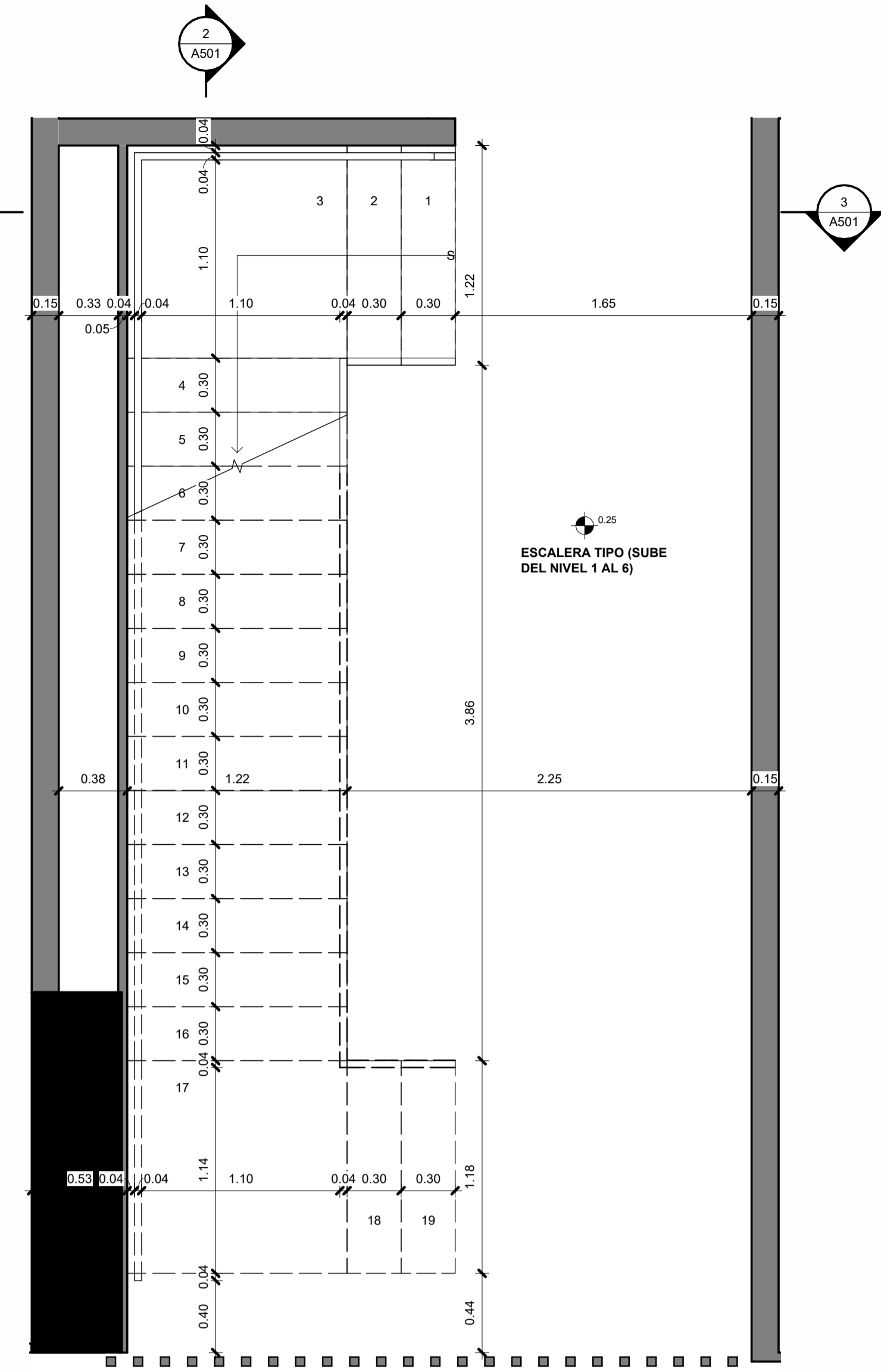
1 Planta Ampliada - Escalera Tipo 1:25
