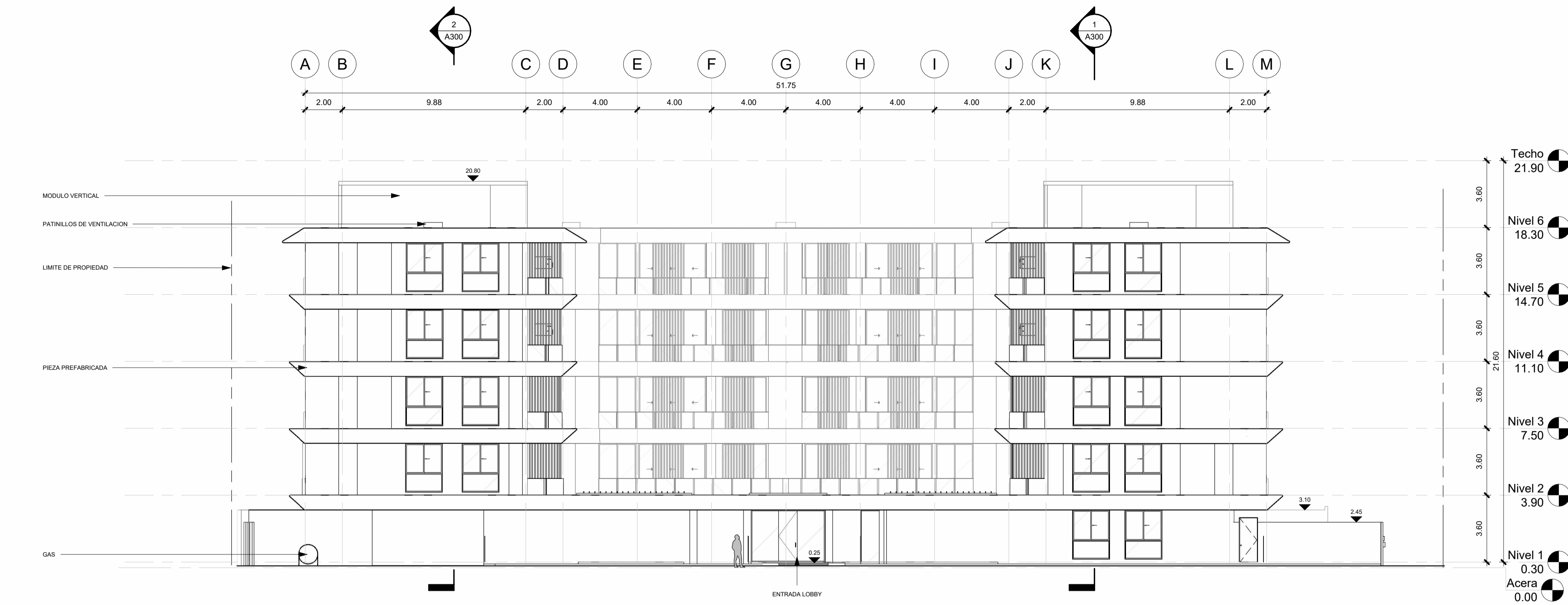
1 Elevación Frontal 1 : 150
