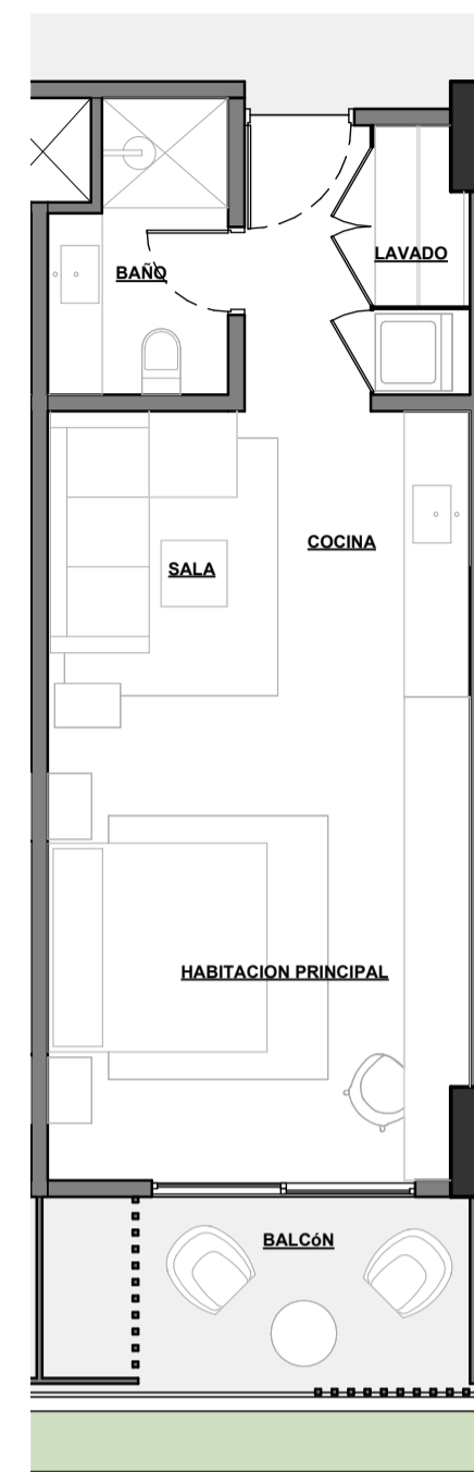
2 Planta Arquitectonica - Tipología A 38M2 1:75
