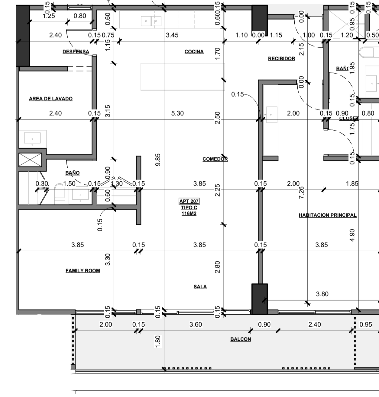
6 Planta Dimensionada - Tipología C 116M2 1:75
