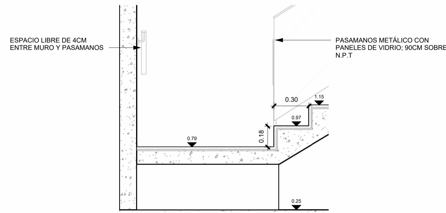
5 Detalle Ampliado de Escalera 2 1:20
