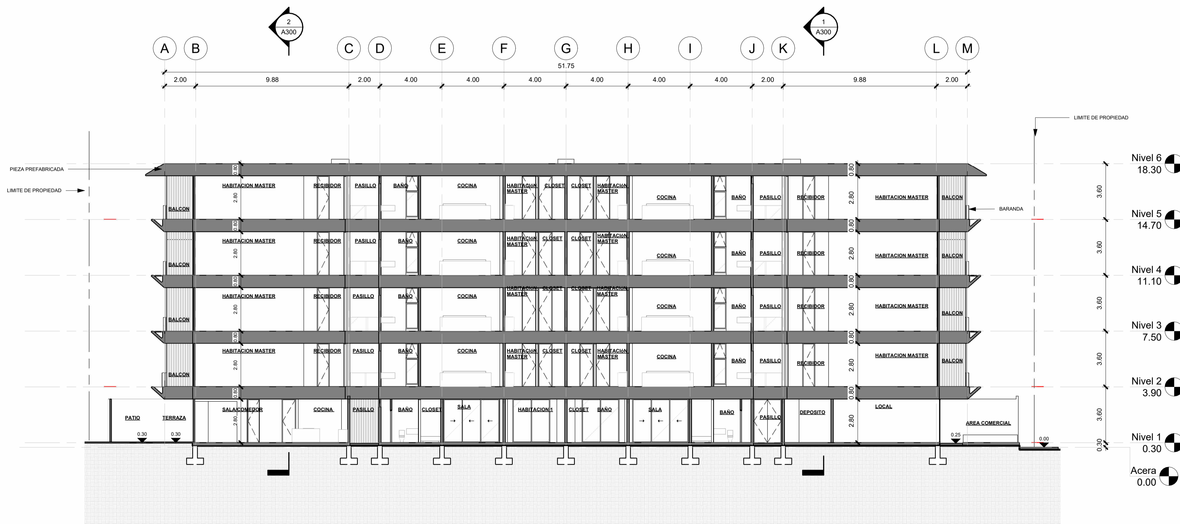
4 Seccion 4 1 : 150
