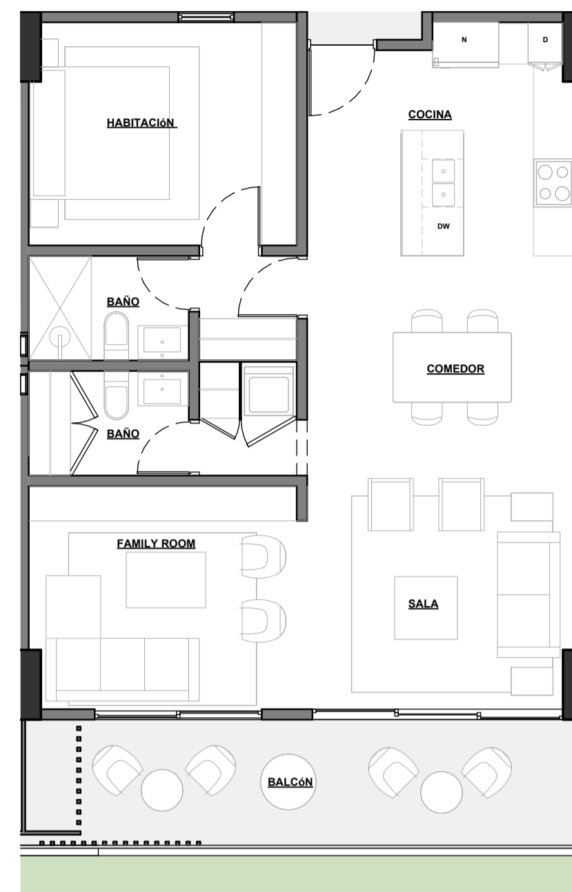
1 Planta Arquitectonica - Tipología B 77M2 1:75
