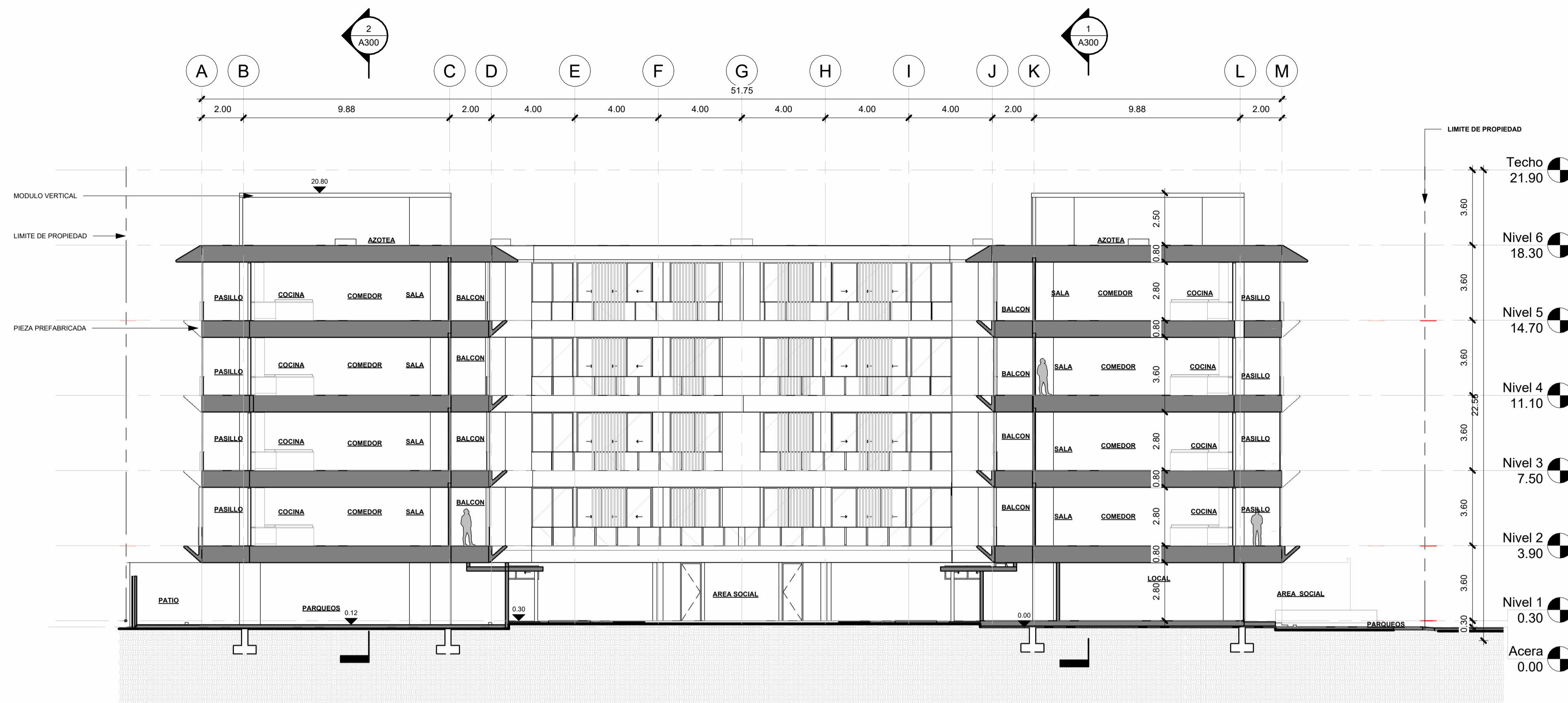
3 Seccion 3 1 : 150
