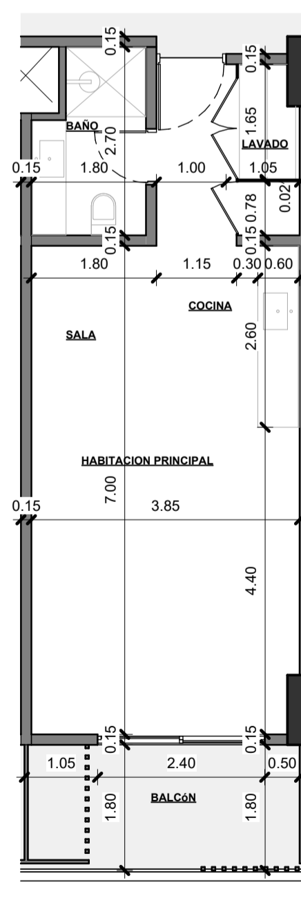
4 Planta Dimensionada - Tipología A 38M2 1:75
