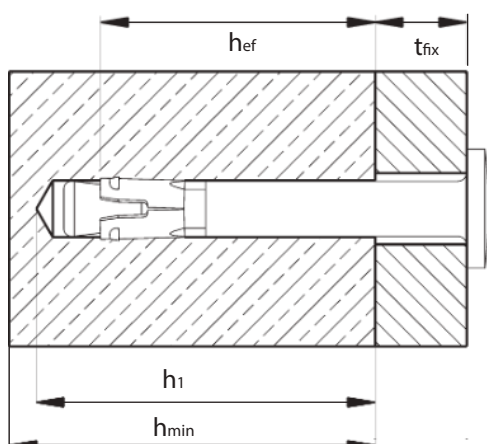
Bild 1: maximale Tragfähigkeit
