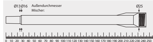
Nutzlänge Statikmischer VM-XL
