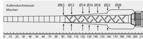
Nutzlänge Statikmischer VM-X
