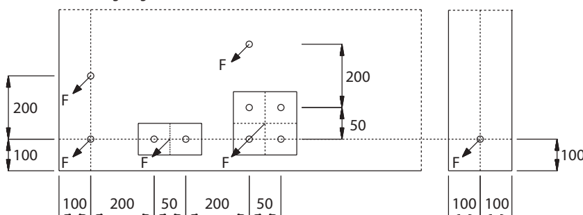
Bild 1: maximale Tragfähigkeit
