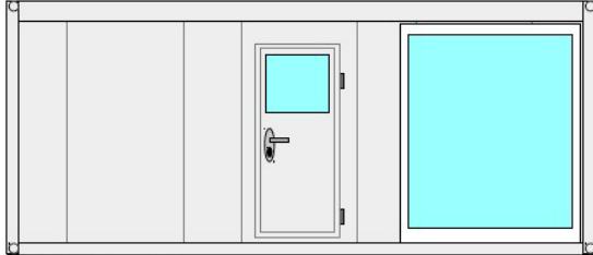
Ansicht Rückseite 1:50
