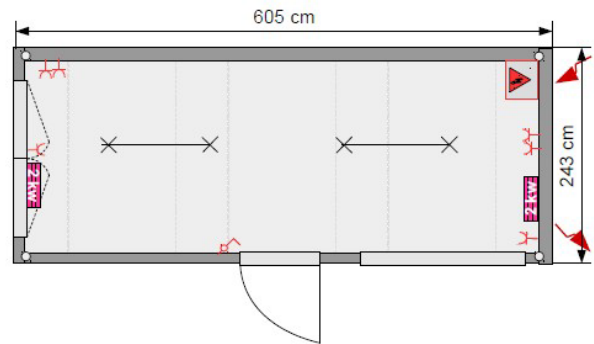
Grundriss 1:50
