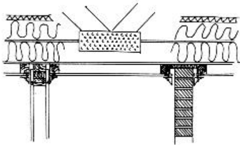
Kuva 11b. Esimerkkejä ei-kantavan väliseinän kiinnityksestä
