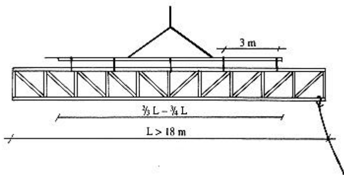
Kuva 8e. Nosto palkin kanssa (ripustettuna viidestä pisteestä)
