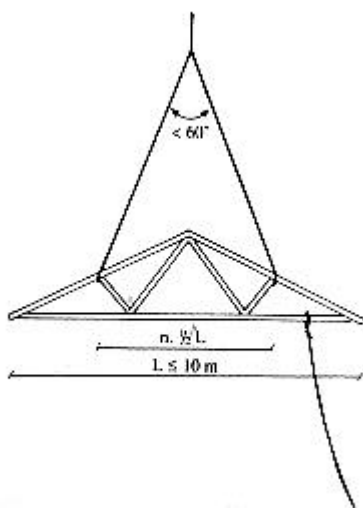
Kuva 8a. Nosto ilman palkkia (harjaristikko)
