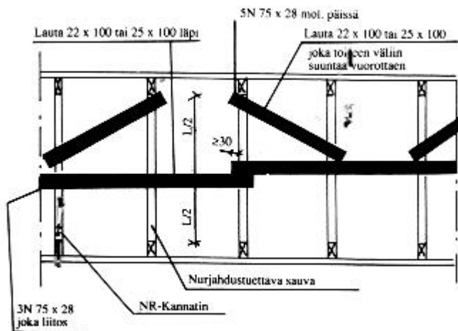
Kuva 12a. Nurjahdustuenta
