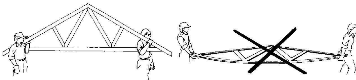
Kuva 2. NR-rakenteiden käsittely
