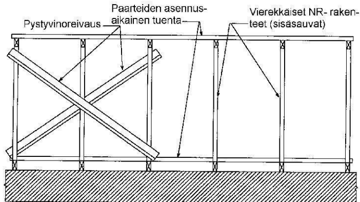
Kuva 8. Asennusaikainen pystyvinoreivaus. X-tukien välinen etäisyys on kannattimen suunnassa enintään 2,5 m.
