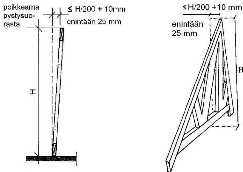
Kuva 7. Pystysuoruuustoleranssi
