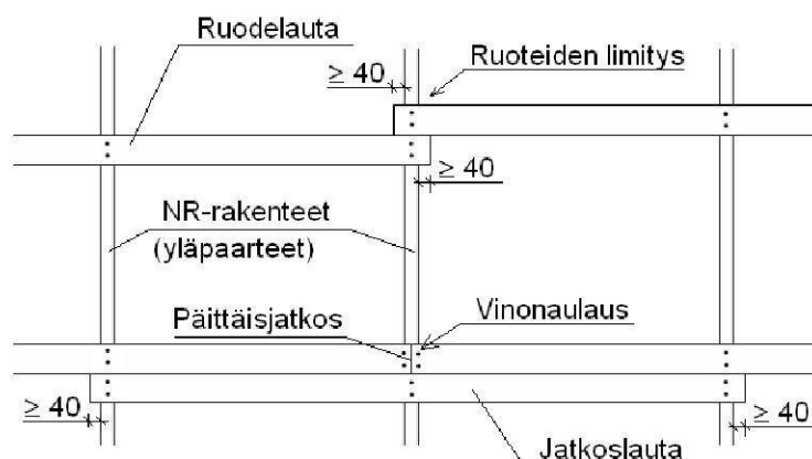
Kuva 15. Ruoteiden limittäminen tai jatkoslaudan käyttö.
