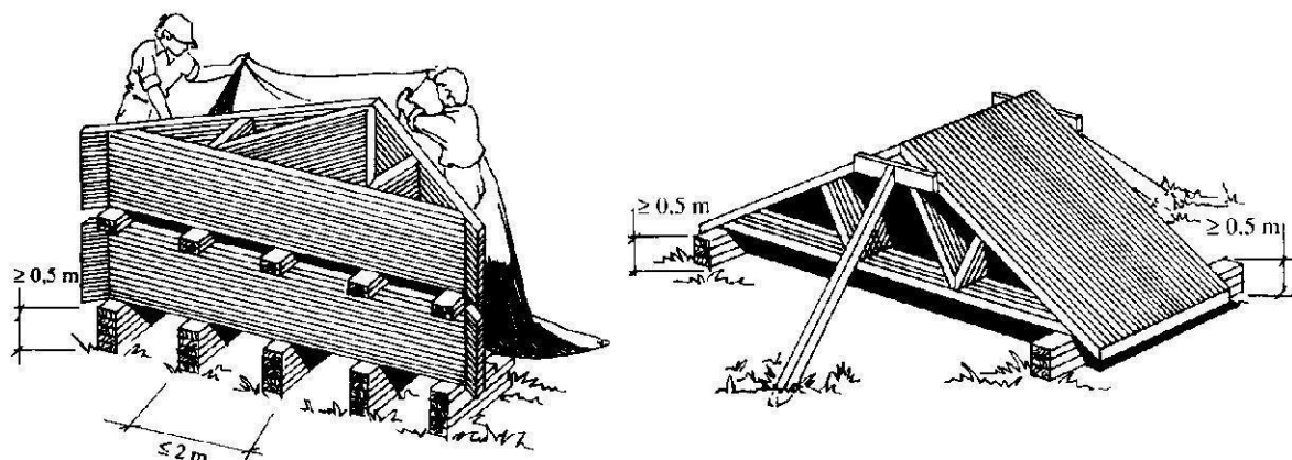
Kuva 1. NR-rakenteiden varastointi.
