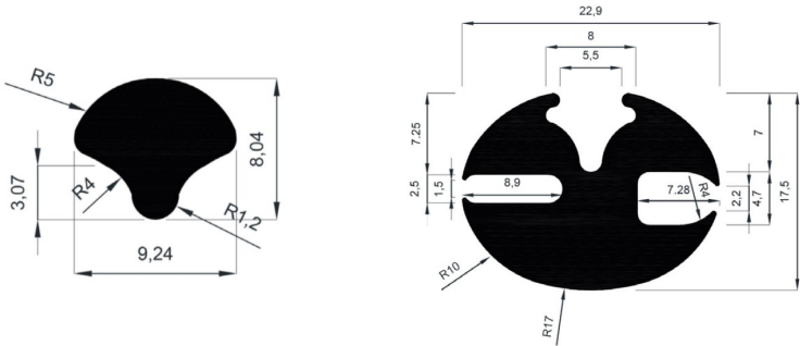
Perfil en caucho EPDM Ref: 105 + junquillo
