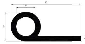
Perfil en caucho EPDM Ref: 19 forma 9
