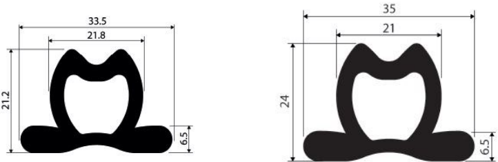
Perfil en caucho EPDM Ref: 14 Y 14G
