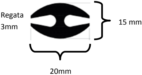
Perfil en caucho EPDM Ref: 13 forma H
