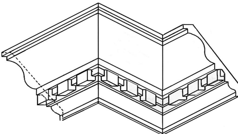
Stuckleiste und Kälberzahnleiste 1302 oder 1303
