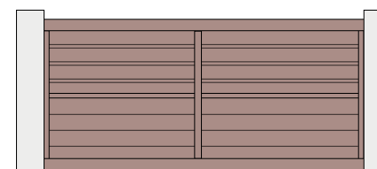
*Lucida C - 6 Lame brise-vent horizontale 150 (haut) Lame pleine horizontale 170 (bas)
