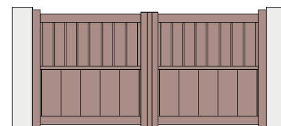
Lucida 2 Lame brise-vent verticale 150 (haut) Lame pleine verticale 255 (bas)
