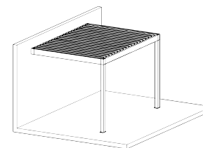
Adossée lames perpendiculaires
