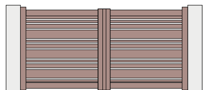
Nordet Remplissage horizontal Lames de 40, 80 et 160 mm
