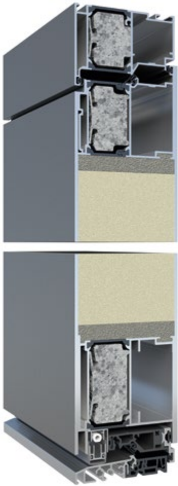
Querschnitt Profilsystem KOtherm 96
