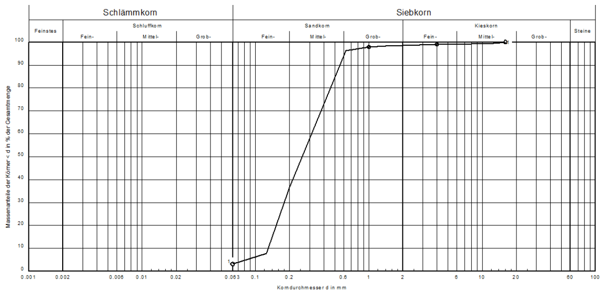
Abbildung 1: Korngrößenverteilung für Siebsand
