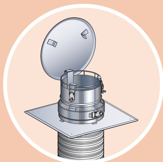
Visuel du chapeau Ø 80-100 intégrant le dispositif anti-oiseau
