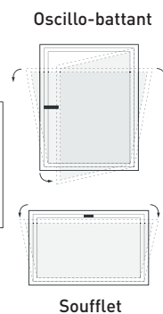
Soufflet
