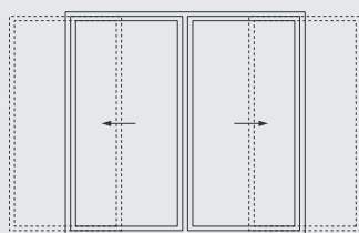
Coulissant à galandage 2 vantaux 1 rail à refoulement opposé
