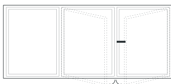
Ensemble composé 3 vantaux dont 1 fixe
