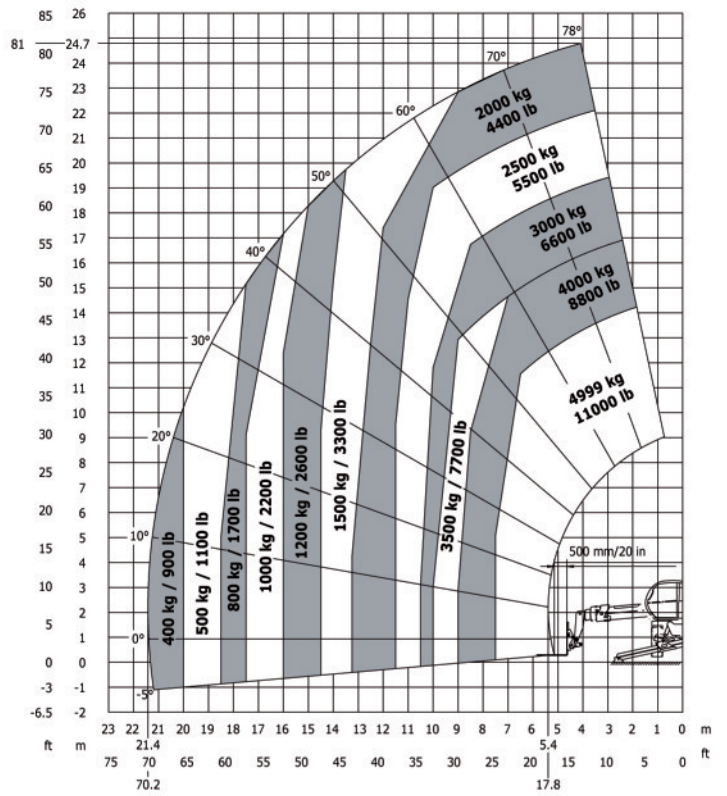
Drehung auf ausgefahrenen Stützen mit Arbeitsbühne 1000
