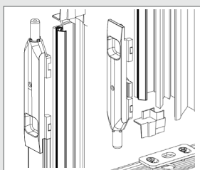
Verrou haut et bas invisibles sur l'ouvrant
