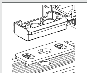
Gâches haute et basse réglables
