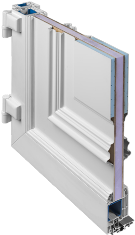
PORTE PVC À PANNEAU UD 1,3*
