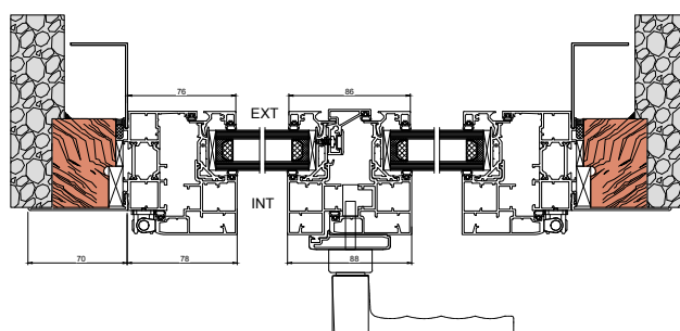
Poignée Rasata
