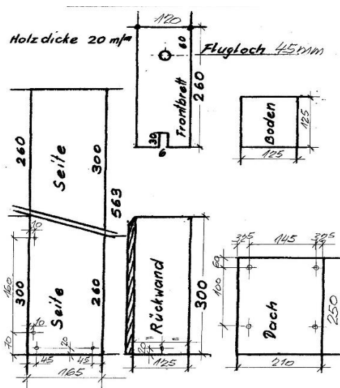
Fabrikationsplan Nistkasten für Stare
