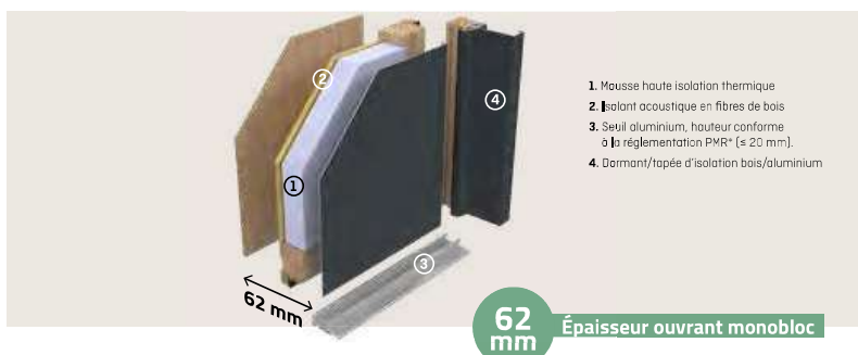
INTÉRIEUR BOIS
