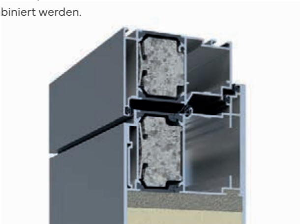
Abb. flügelüberdeckende Füllung innen und außen
