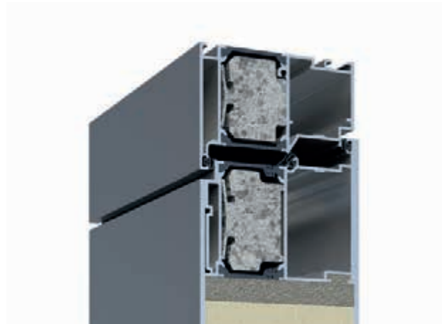
Abb. flügelüberdeckende Füllung innen und außen
