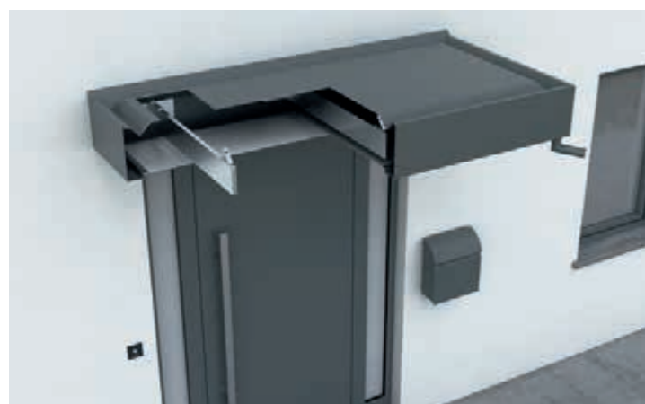
Tragarmkonstruktion z.B. Vordach Typ KV 380 Die Anzahl der Tragarme richtet sich nach der Größe des Vordaches (ohne Befestigungsmaterial).
